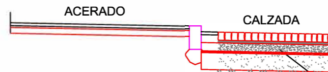
SECCIÓN ACTUACIÓN AA'
